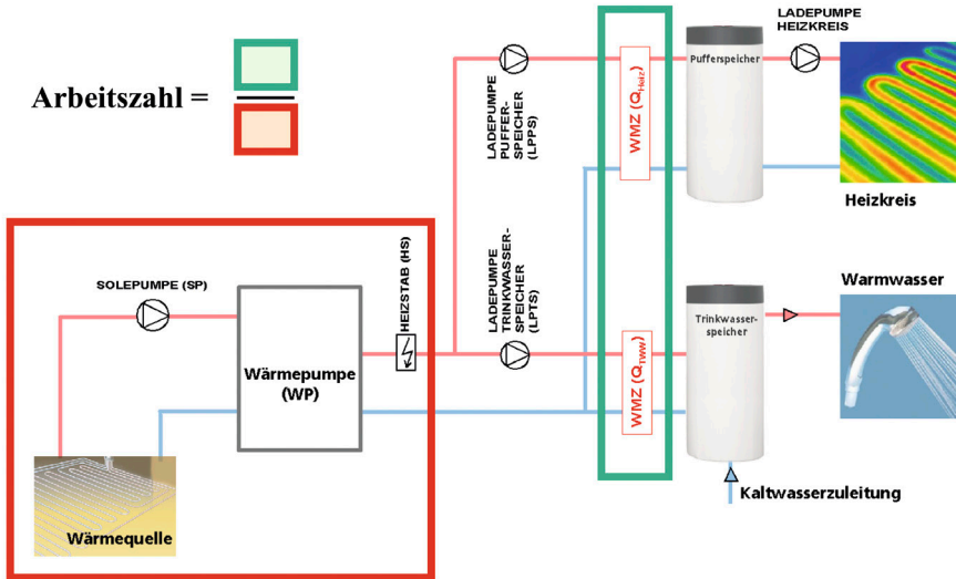
Abb. 9: Schematische Darstellung einer Wärmepumpenanlage mit eingezeichneten Bilanzgrenzen.
